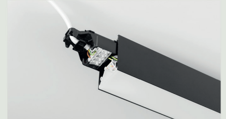
2 | zugängliches Kabelfach
